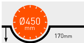
PROFONDEUR DE COUPE MAXI. CS451 E
